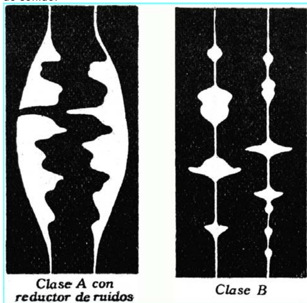
Figura 123. Bandas Push-Pull
