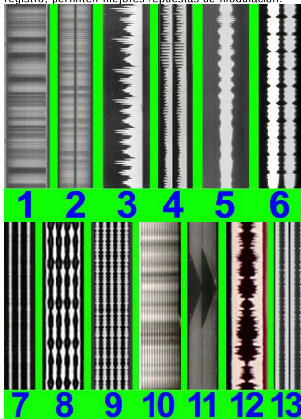
Figura 120. Clasificación morfológica de bandas ópticas 1 - Densidad variable (tipo: Western Electric). 2 - Doble Densidad variable (16mm). 3 - Área variable unilateral (Tipo: RCA). 4 - Doble unilateral (16mm). 5 - Área variable bilateral simétrica (Tipo: RCA). 6 - Área variable bilateral simétrica bipista (Tipo: British Acoustic). 7 - Tres pistas bilaterales simétricas (16mm). 8 - Área variable multipista (Tipo: MGM 5 pistas). 9 - Área variable multipista (Tipo: Tobis KlanFilm 7 pistas). 10 - Área variable multipista (Tipo: Laffon-Selgas 14 pistas). 11 - Doble multipista (16mm). Este ejemplo presenta un doble silenciador en empalme). 12 - Área variable Duplex. 13 - Área variable doble Duplex (16mm)
