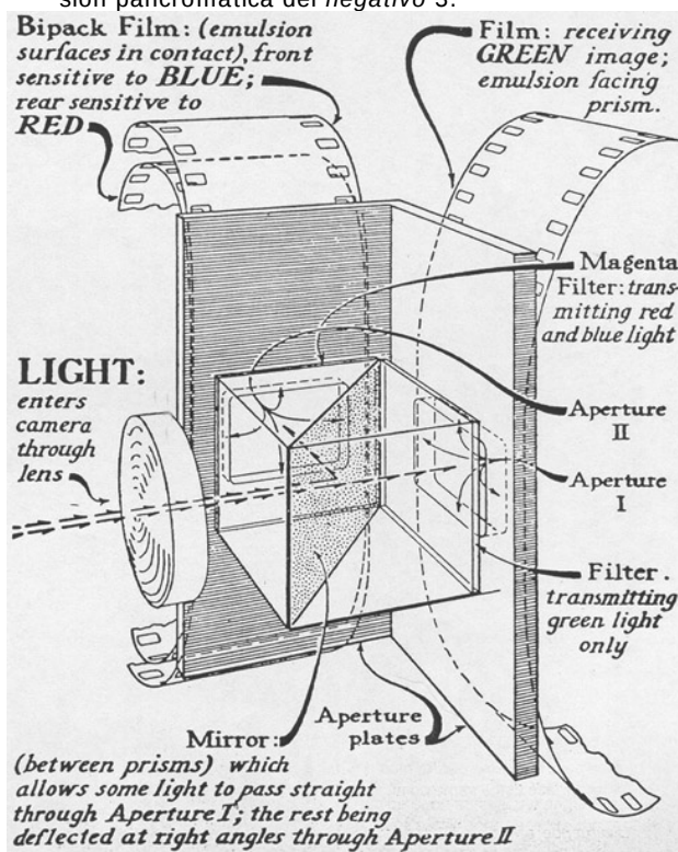
Figura 42. Sistema de filmación en Technicolor (Ilustración de "American Cinematographer", VIII – 1981, pg.792)
