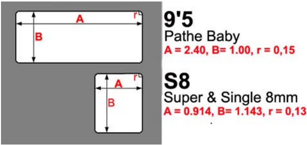
Figura 92 Perforaciones estandarizadas para 9'5 y Super 8mm. La perforación de las películas de 8mm (Doble 8) es idéntica a las del paso 16mm.
