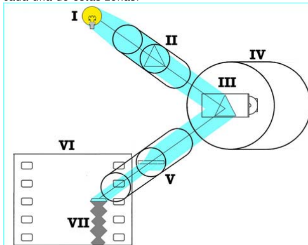
Figura 118. Esquema de un sistema de densidad variable (Siguiendo el esquema desarrollado por la RCA)
