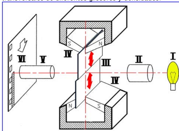
Figura 117. Esquema del sistema de densidad variable
