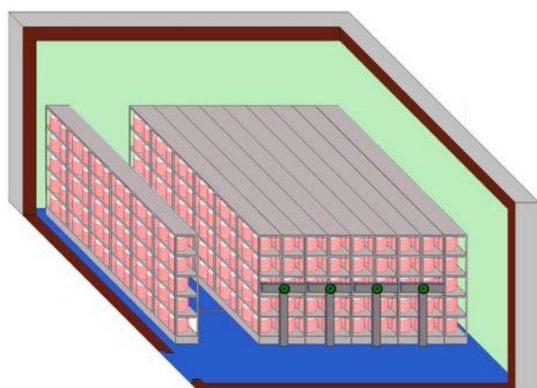
Figura 183. Esquema de almacén con estanterías móviles compactables separadas de la pared.
