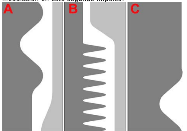
Figura 122. Funcionamiento de los reductores de ruido en bandas de área variable. (Esquema basado en el funcionamiento de las bandas unilaterales).
